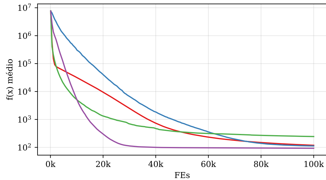
Rastrigin — D=100
