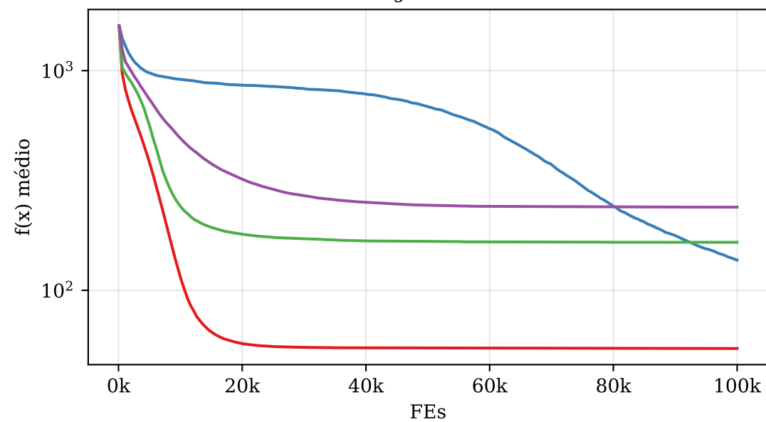
Schwefel 2.26 — D=100
