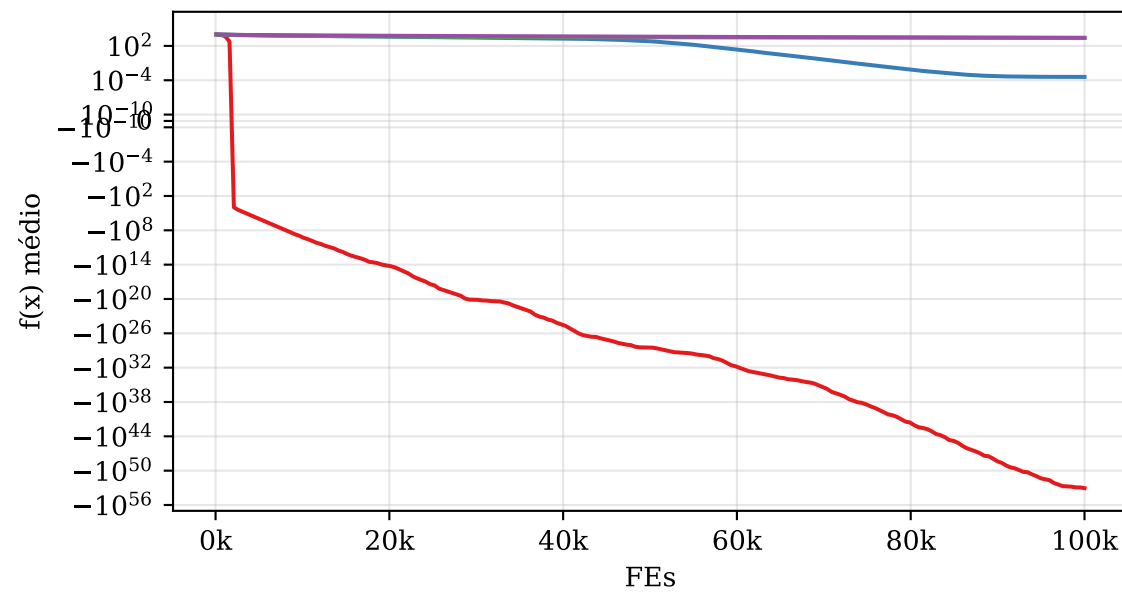
Schwefel 2.26 — D=30
