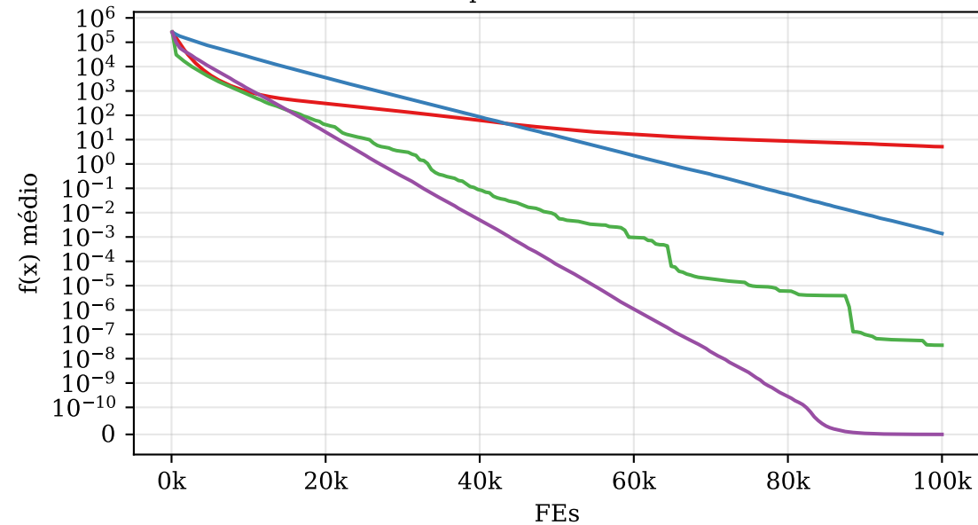
Rosenbrock — D=100
