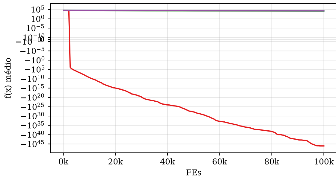
Schwefel 2.26 — D=100
