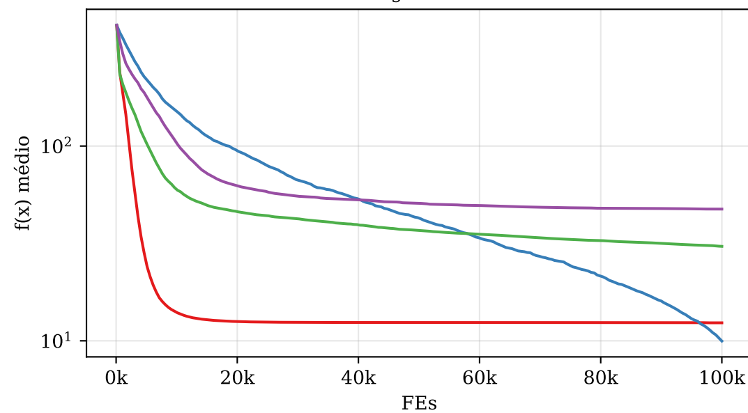
Schwefel 2.26 — D=30
